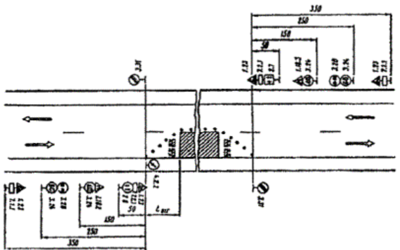
Рис. 3.2. Организация движения и ограждение места дорожных работ, выполненных на половине ширины проезжей части двухполосных дорог
