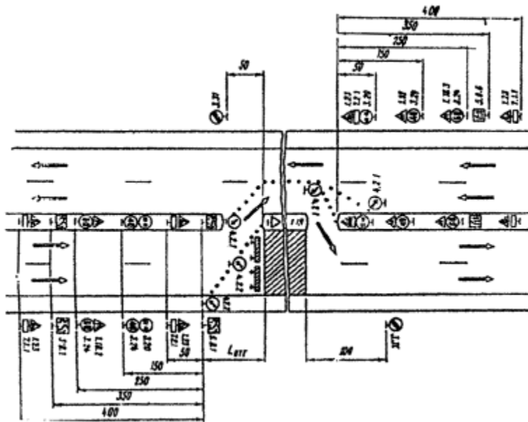
Рис. 3.7. Организация движения и ограждение мест дорожных работ, выполняемых на разделительной полосе многополосных дорог
