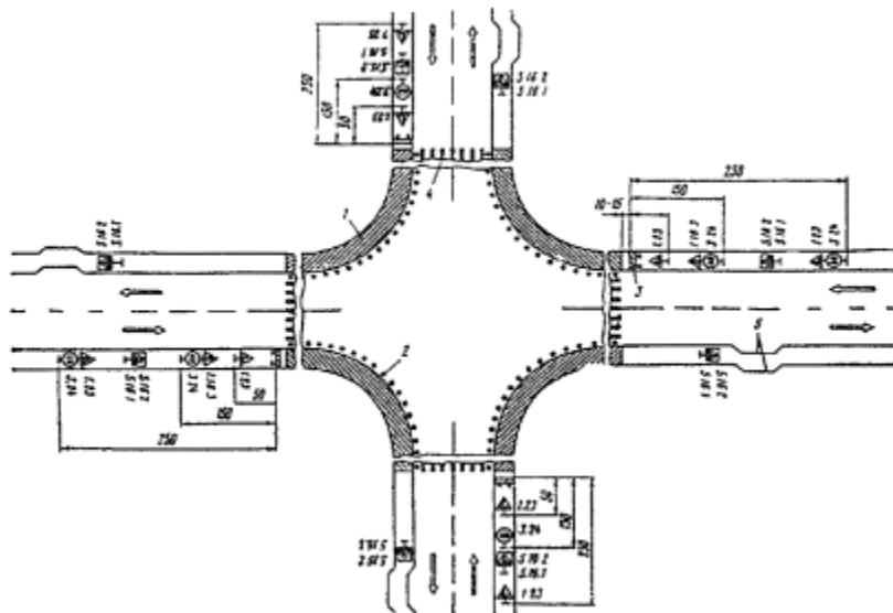
Рис. 3.14. Организация движения и ограждение мест дорожных работ, выполняемых на обочинах пересечения в одном уровне:
