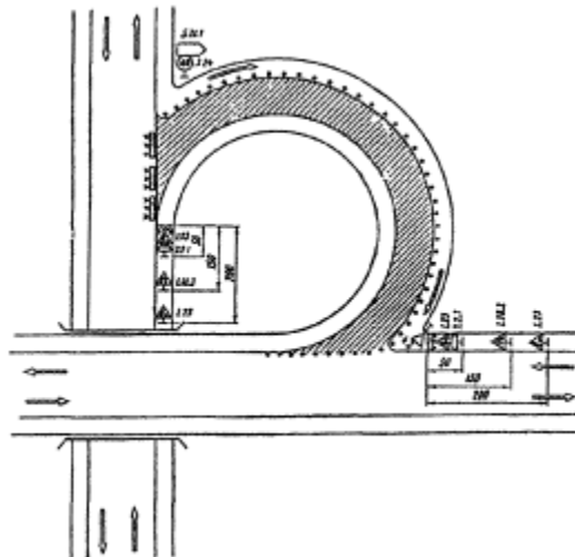
Рис. 3.19. Организация движения по обочине и ограждению места дорожных работ, выполняемые на всей ширине проезжей части правоповоротного съезда пересечения в разных уровнях
