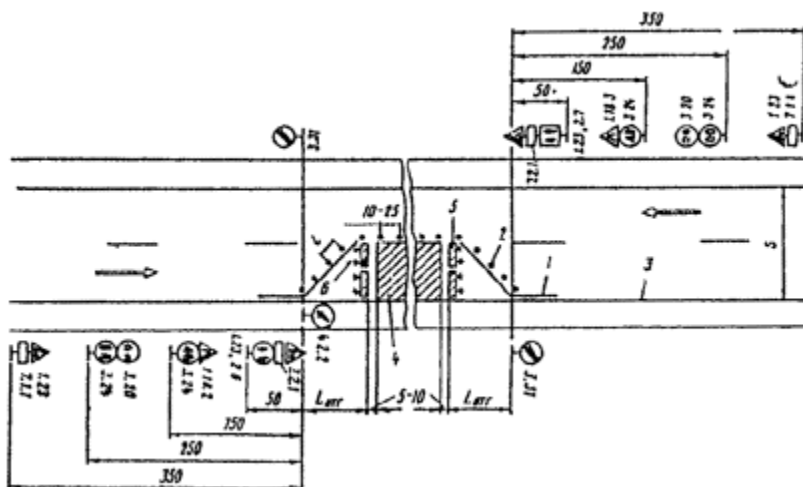
Рис. 2.1. Пример размещения технических средств организации движения в местах производства дорожных работ:
