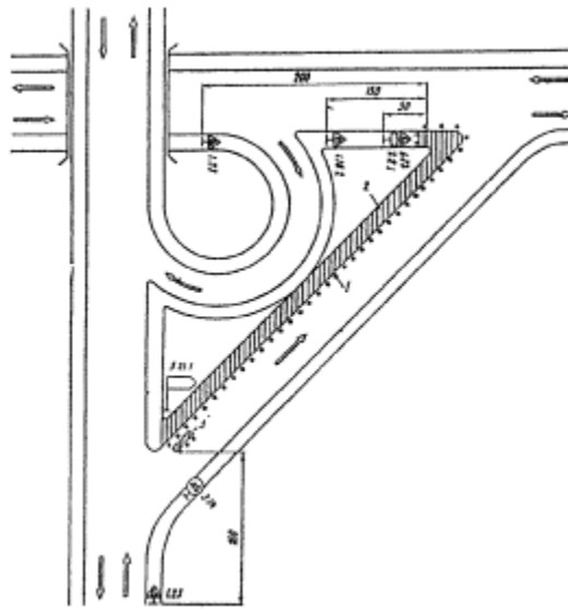
Рис. 3.17. Организация движения и ограждение места дорожных работ, выполняемых на внутренней обочине правоповоротного съезда пересечения в разных уровнях:
