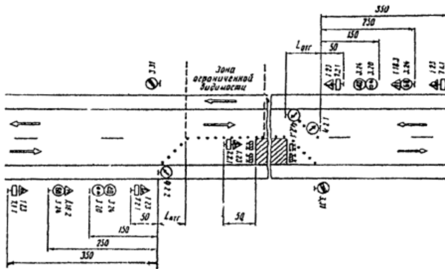
Рис. 3.13. Организация движения и ограждение места дорожных работ на участках с ограниченной видимостью
