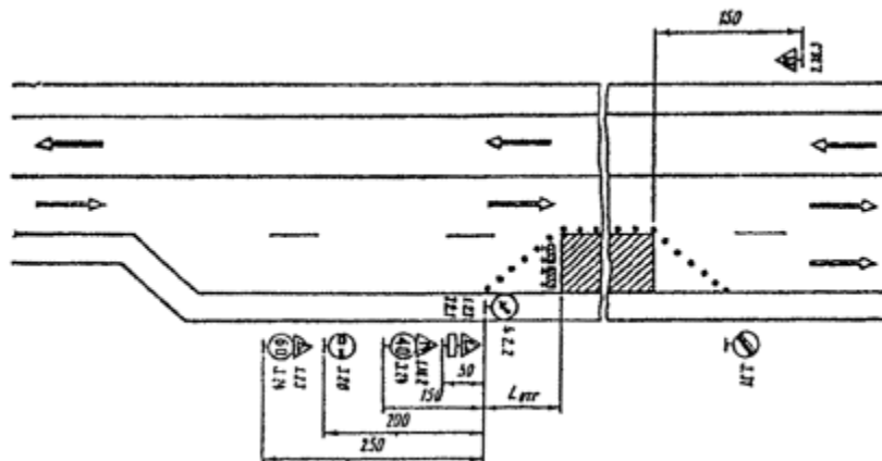
Рис. 3.10. Организация движения и ограждение места дорожных работ, выполняемых на дополнительной полосе на подъеме
