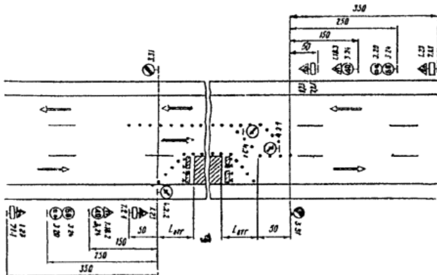
Рис. 3.3. Организация движения и ограждение места дорожных работ, выполняемых на половине ширины проезжей части двухполосных дорог в случае пропуска транспортных средств по обочине
