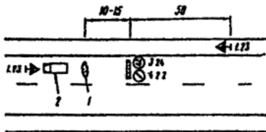
Рис. 3.33. Организация движения и ограждение зоны краткосрочных дорожных работ, вызывающих сужение проезжей части:
