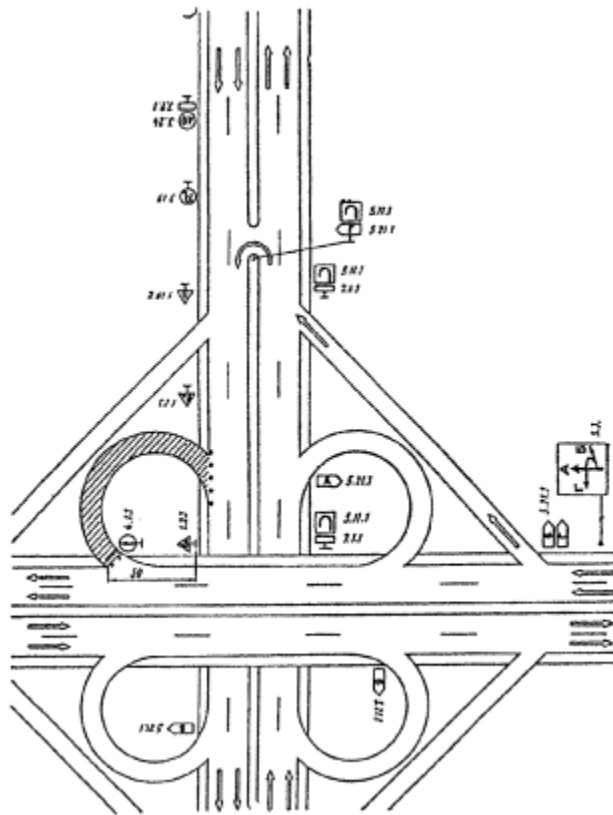
Рис. 3.22. Организация движения и ограждение места дорожных работ, выполняемых на всей ширине проезжей части левоповоротного съезда пересечения в разных уровнях
