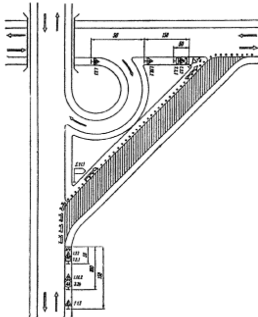
Рис. 3.18. Организация движения и ограждение места дорожных работ, выполняемых на внешней обочине левоповоротного съезда пересечения в разных уровнях
