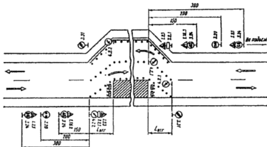
Рис. 3.9. Организация движения и ограждение места дорожных работ в случае уширения проезжей части на участках, затяжных подъемах двухполосных дорог
