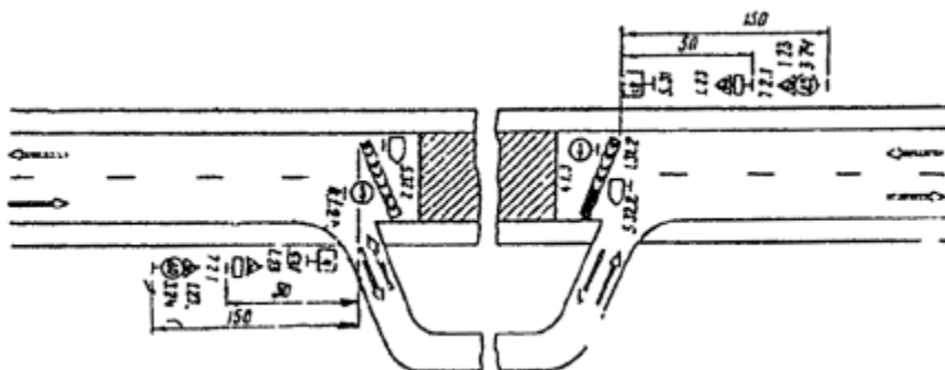
Рис. 3.30. Организация движения при производстве дорожных работ на всей ширине проезжей части и направлением потока транспорта в объезд по существующим дорогам
